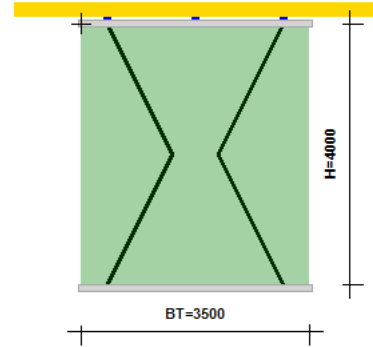
Ankergrund 50 % ueberhoeht dargestellt !
