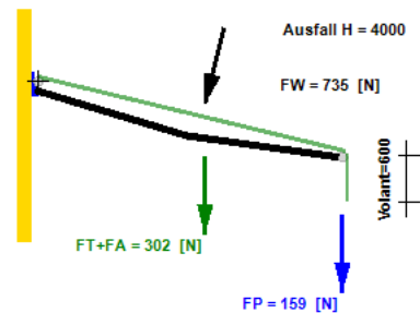
neigm Neigung der Markise = 14 grad
